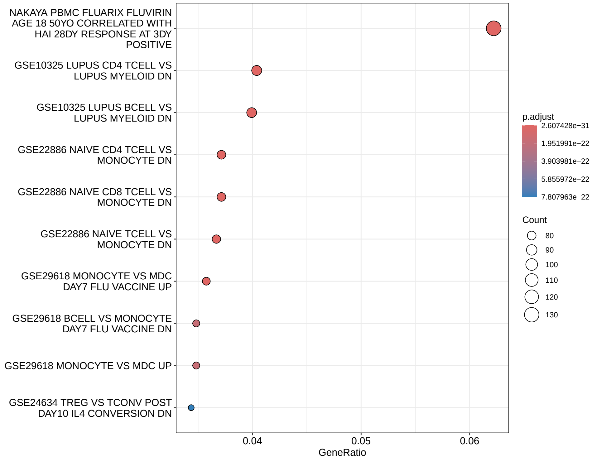
TTL4kd – ORA Dotplot
